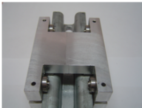
Bild Nr.4 Prüflehre über die gesamte Länge des Profils ziehen.
