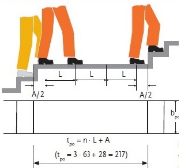
Bild 2: Podesttiefe in Abhängigkeit vom Gangrhythmus
