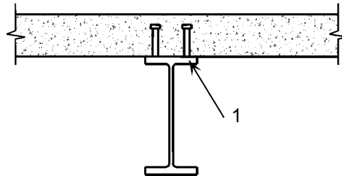
Bild 6.5 — Beispiel für eine Verdrehungsbehinderung
