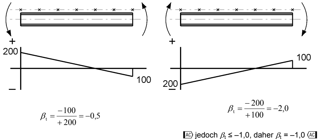
Bild BB.4 — Bestimmung von \beta_t
