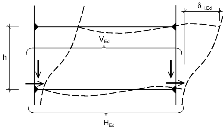
Bild 5.1 — Bezeichnungen zu 5.2.1(4)
